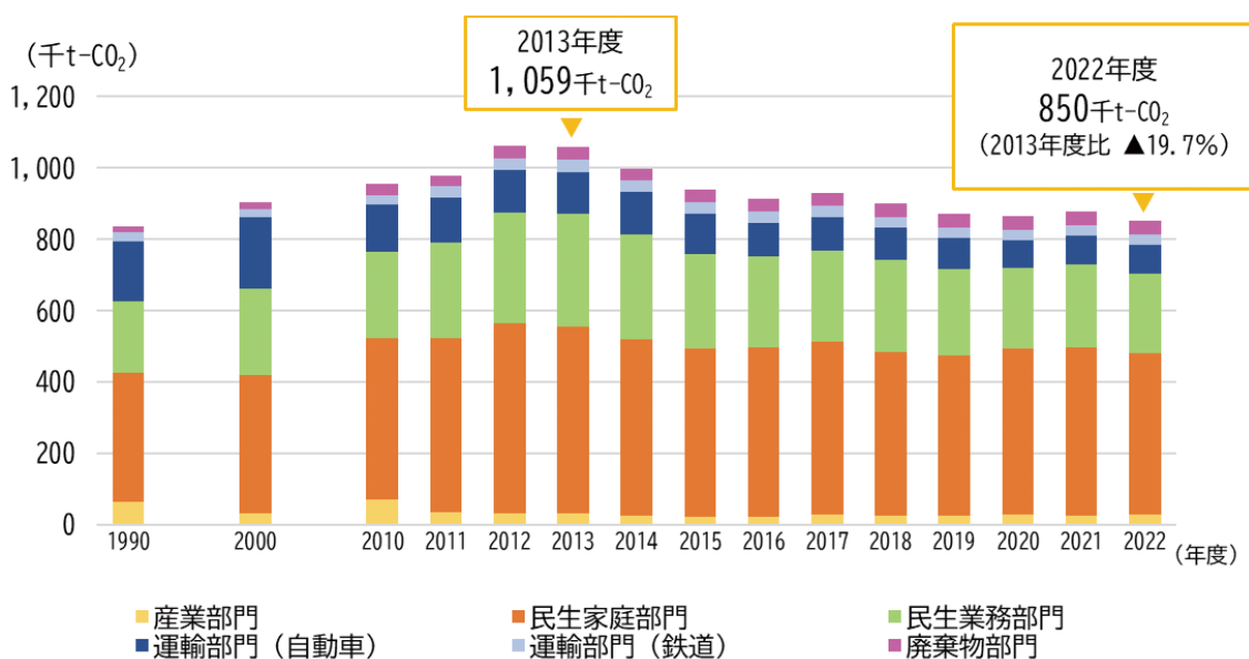
二酸化炭素排出量の推移
