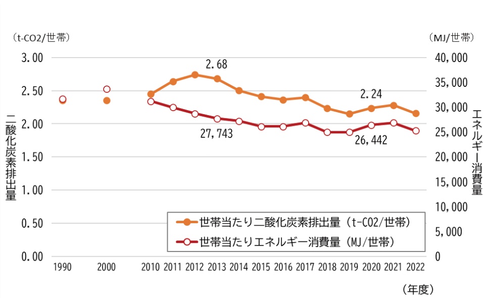
世帯当たりの二酸化炭素排出量とエネルギー消費量の推移
