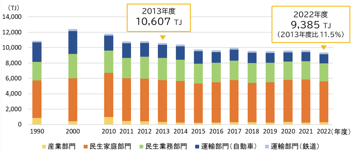
エネルギー消費量の推移
