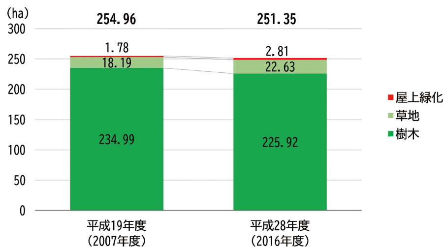
緑被面積の変化
