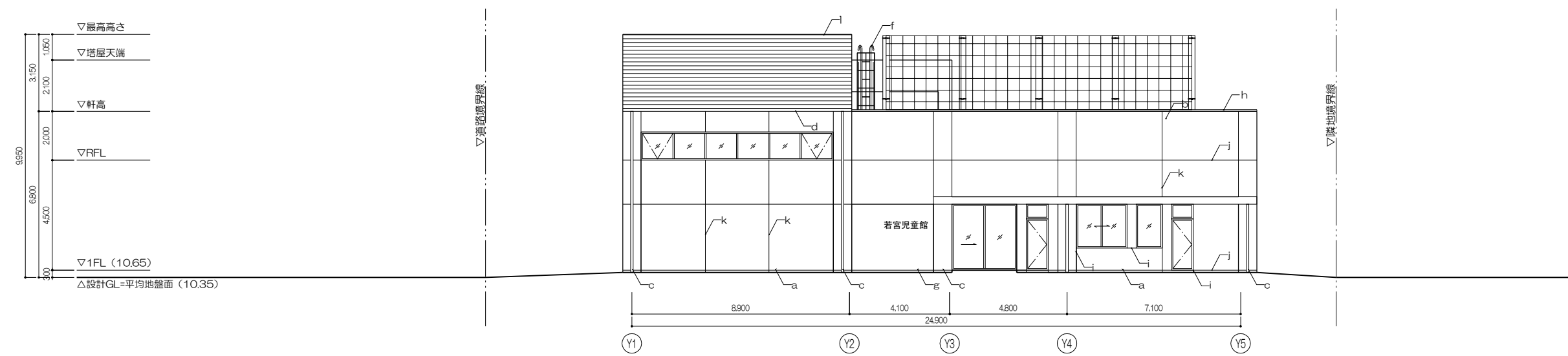
東立面図
