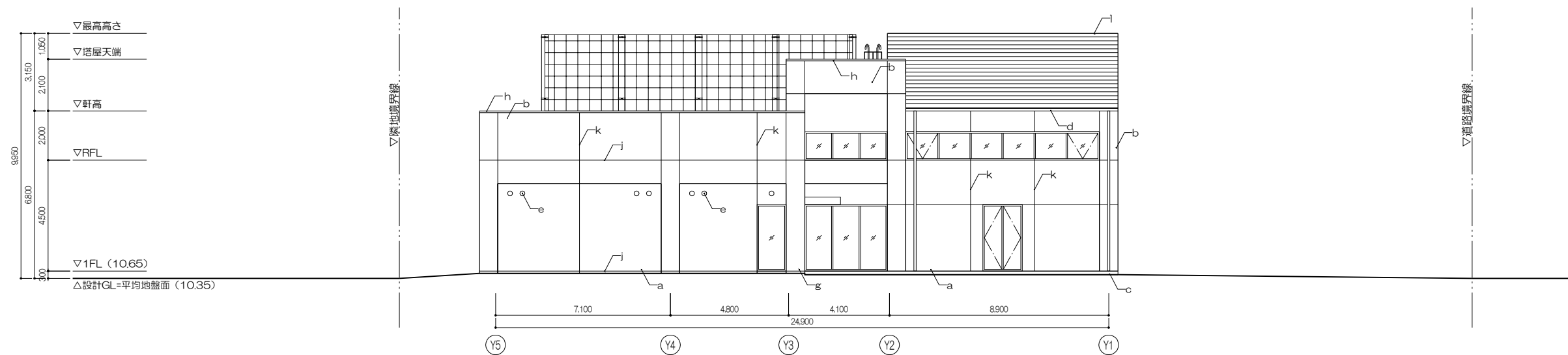
西立面図
