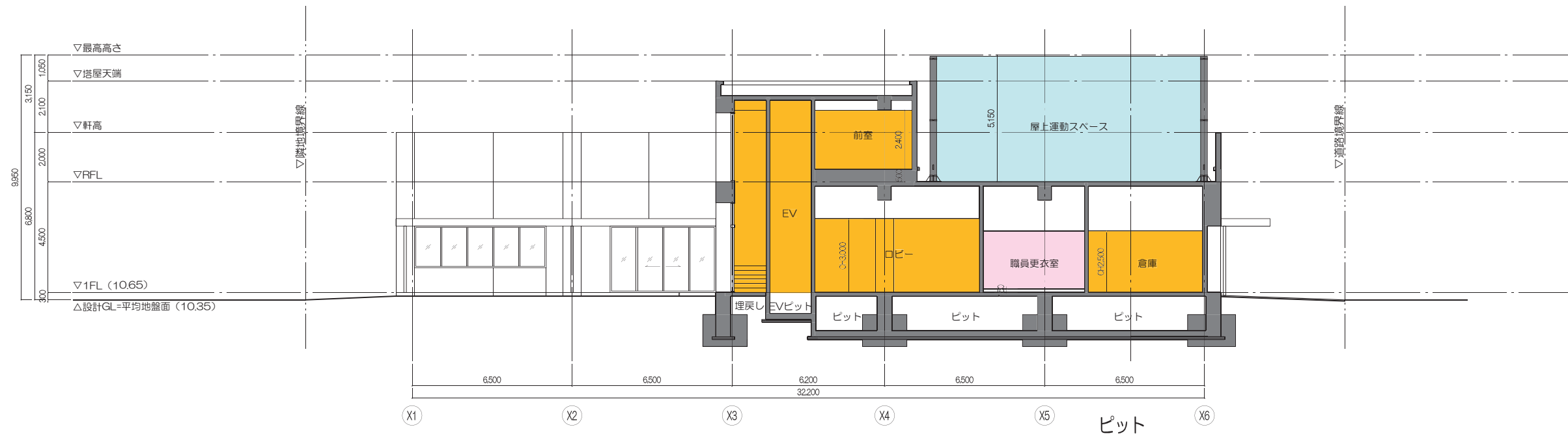
A-A' 断面図
