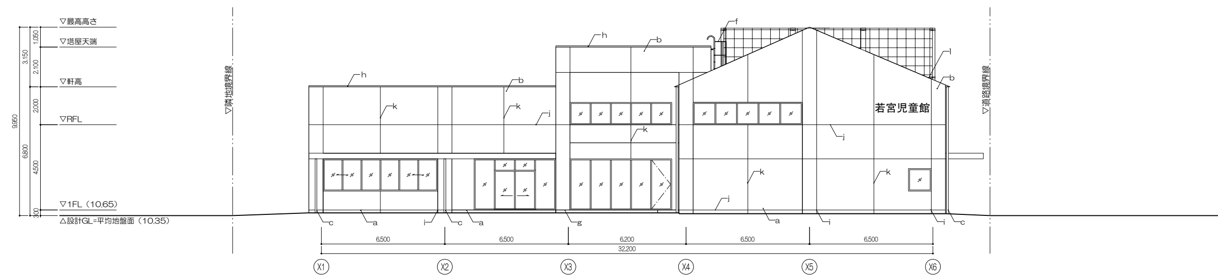
南立面図
