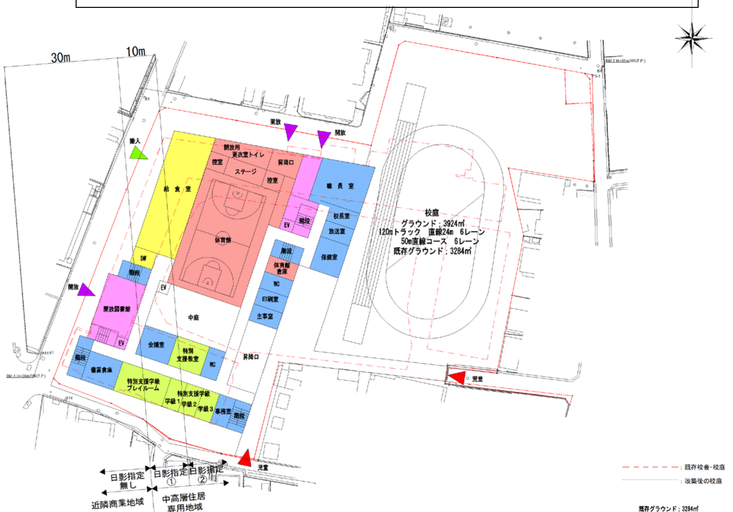
1階平面図兼配置図 (S=1/1000)
