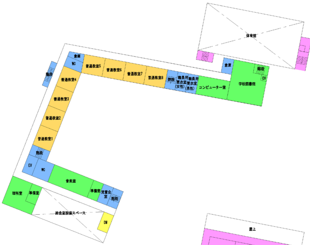
2階平面図 (S=1/1000)
