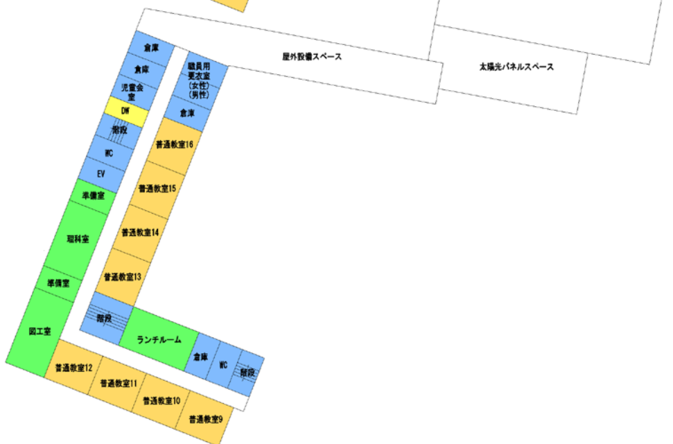
3階平面図 (S=1/1000)
