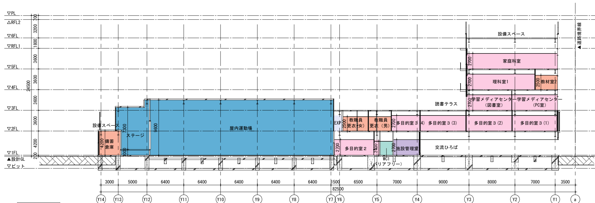
B-B' 断面図
