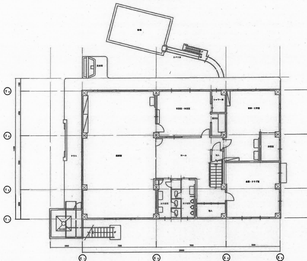
文園児童館 1階平面図 S=1/50
