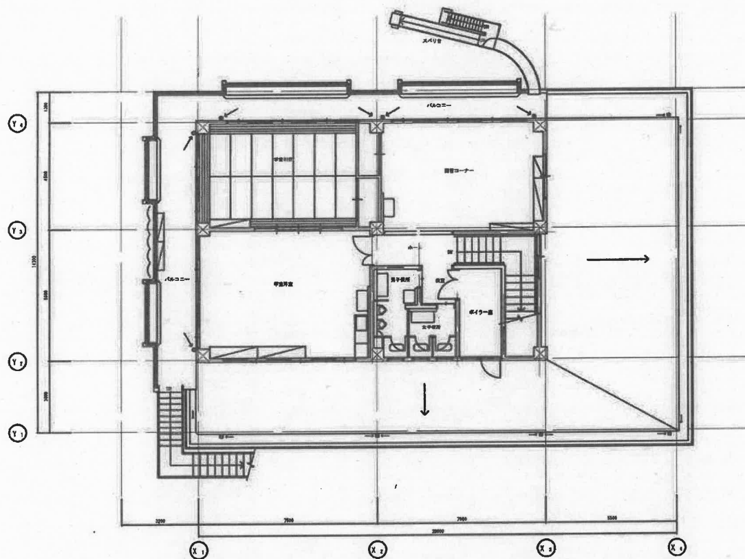
文園児童館及び桃園第二学童クラブ 2階平面図 S=1/50
