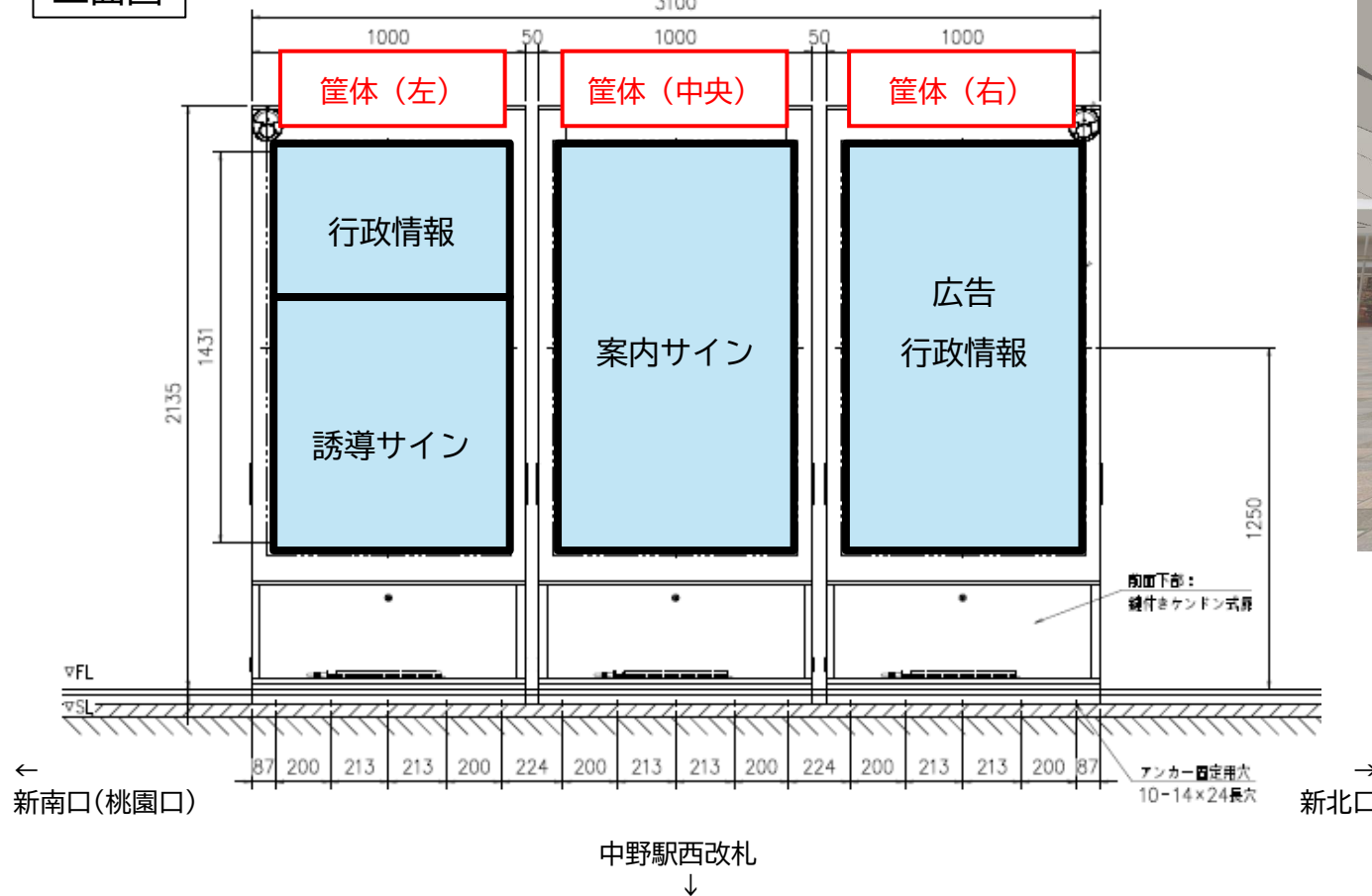
立面図
