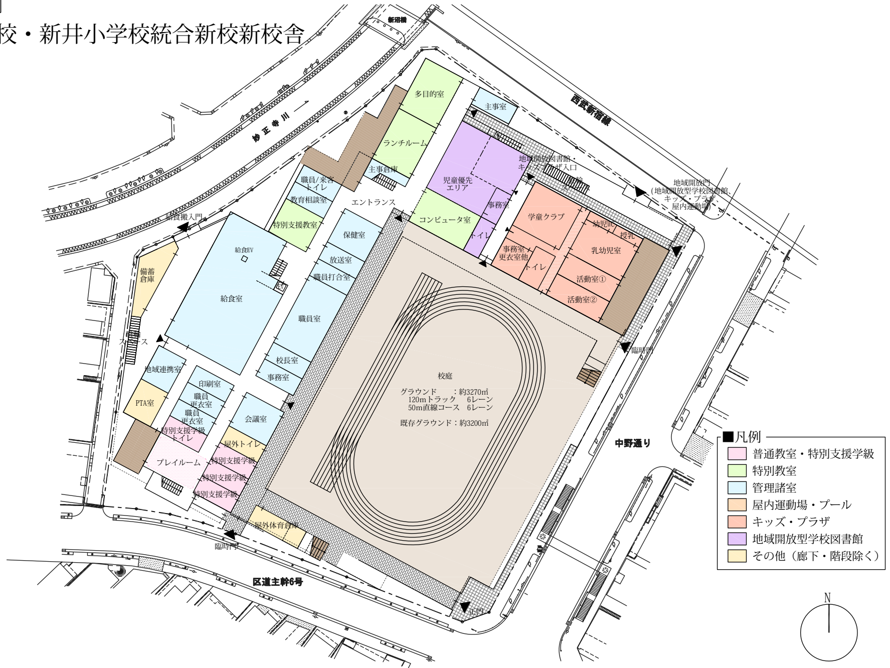
1階平面図兼配置図 (S=1/800)
