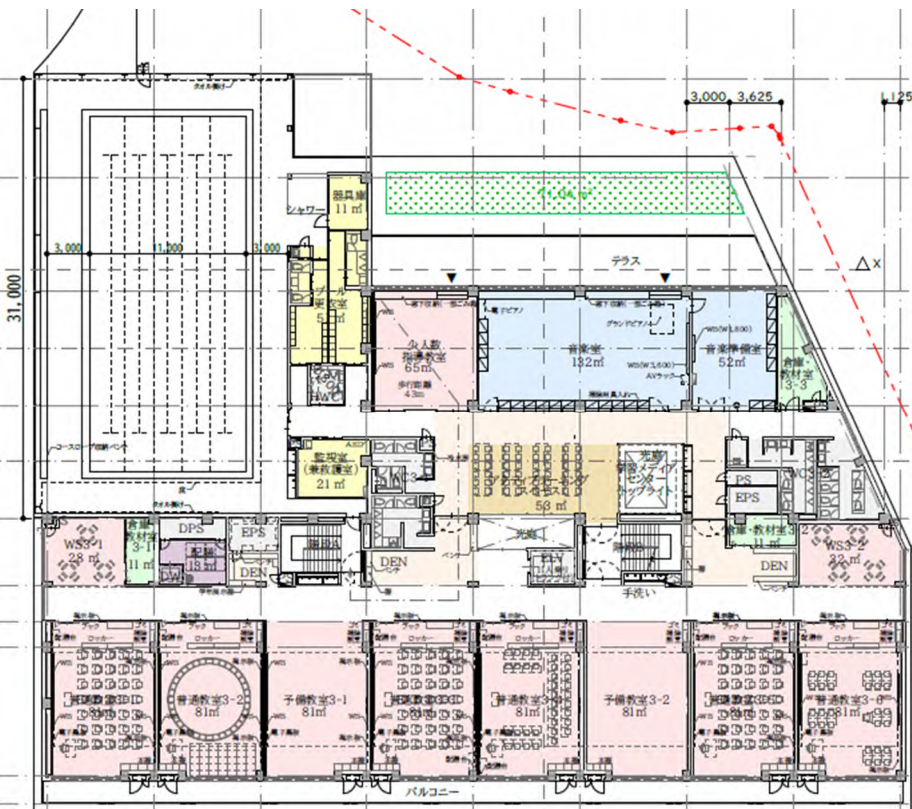
かいへいめんず 3階平面図
