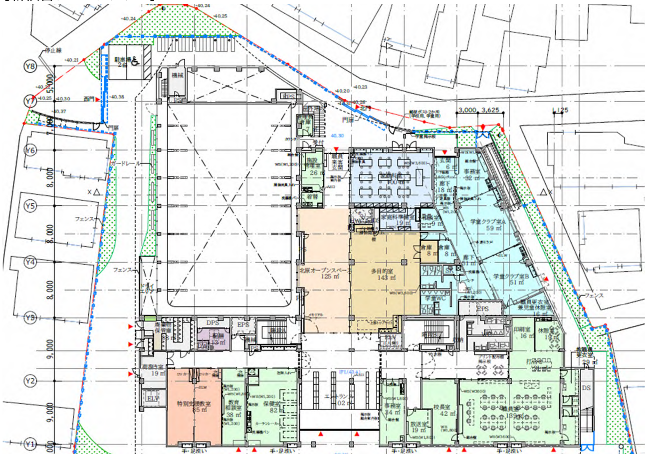
1階配置図(校舎)
