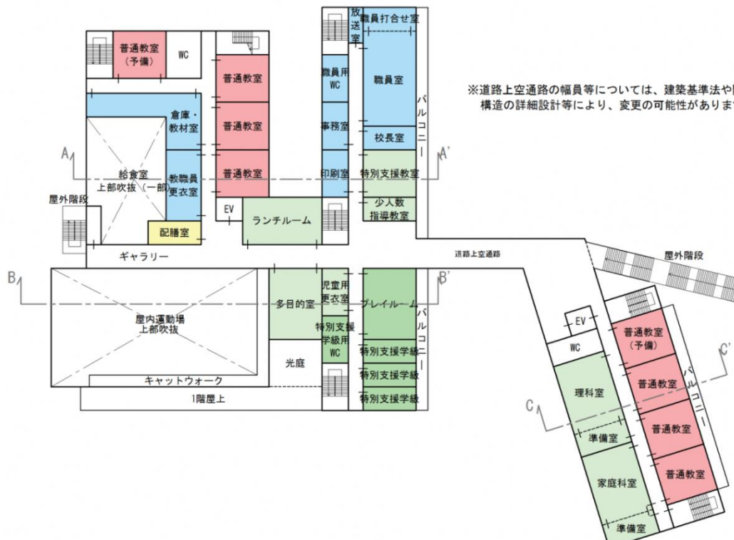
北側敷地2階・南側敷地3階平面図
