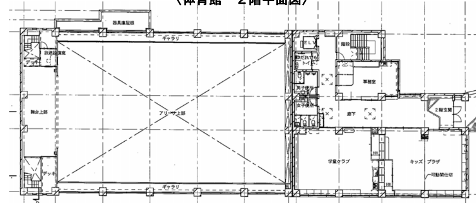
〈体育館 2階平面図〉
