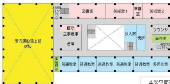
4階平面図
