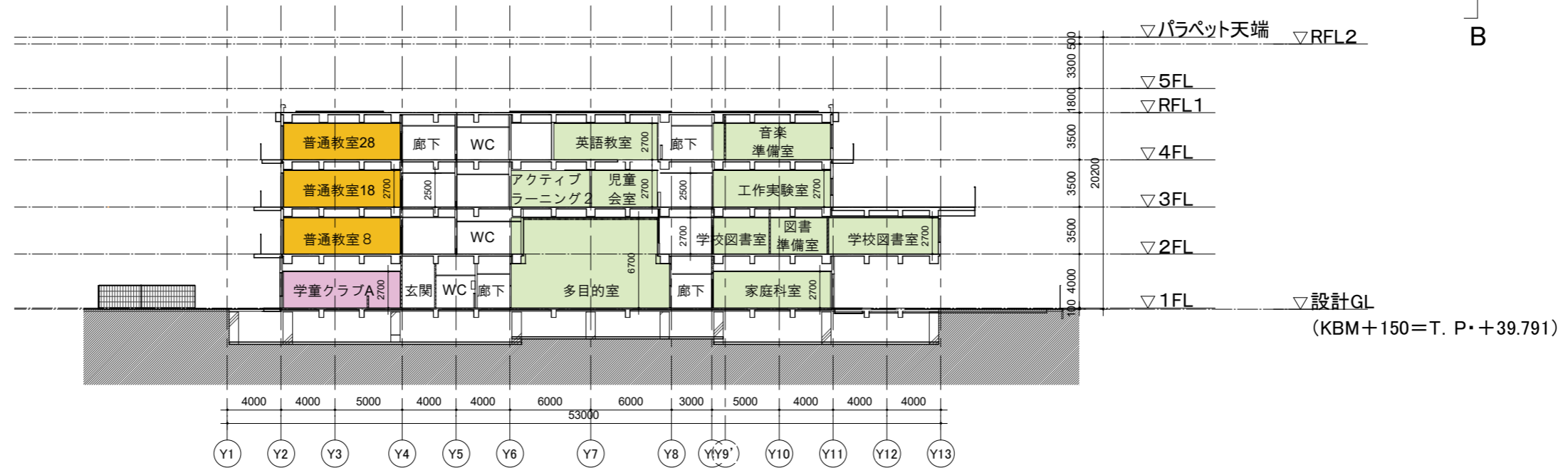
C-C' 断面図
