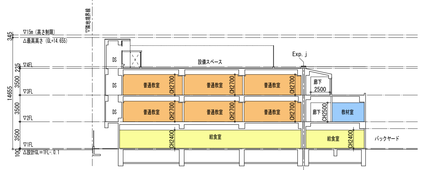
○ Bb-Bb' 断面図
