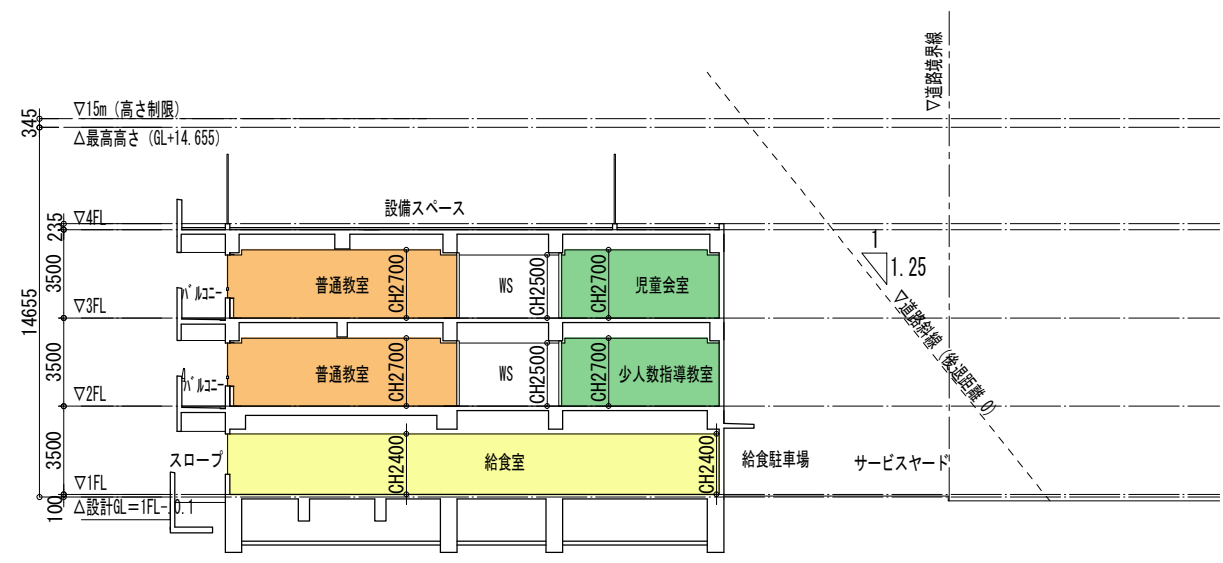
○ Ba-Ba' 断面図
