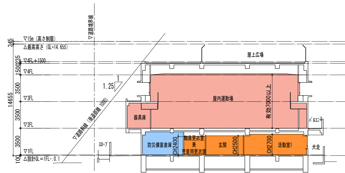
○ Ca-Ca' 断面図
