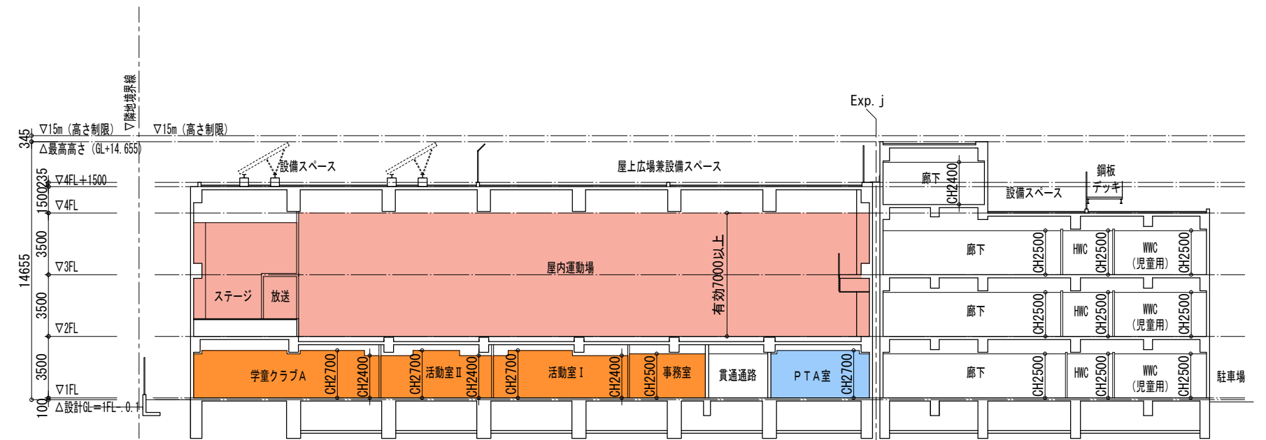
○ Cb-Cb' 断面図
