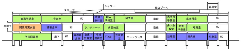
C-C' 断面図(S=1/800)
