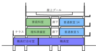
A-A' 断面図(S=1/800)
