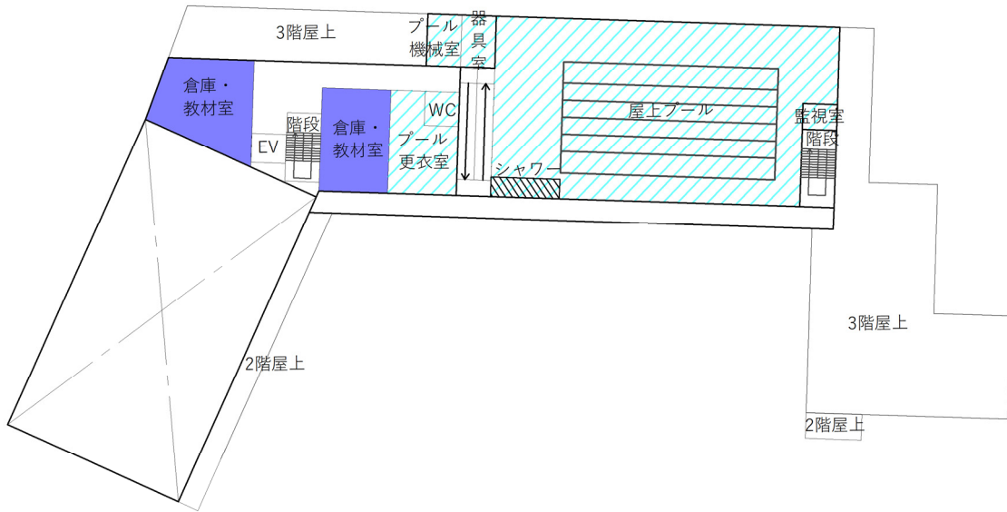
4階平面図 (S=1/800)
