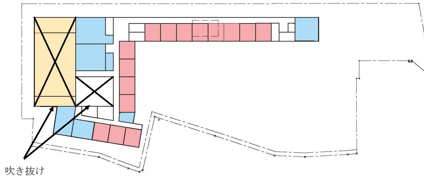
2階平面図
